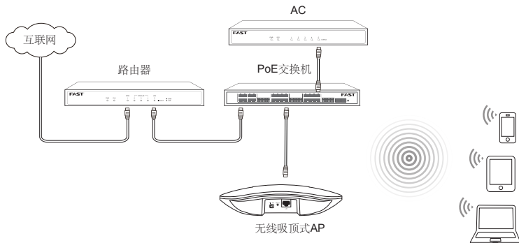
图1-4 典型应用拓扑图-FIT AP模式
