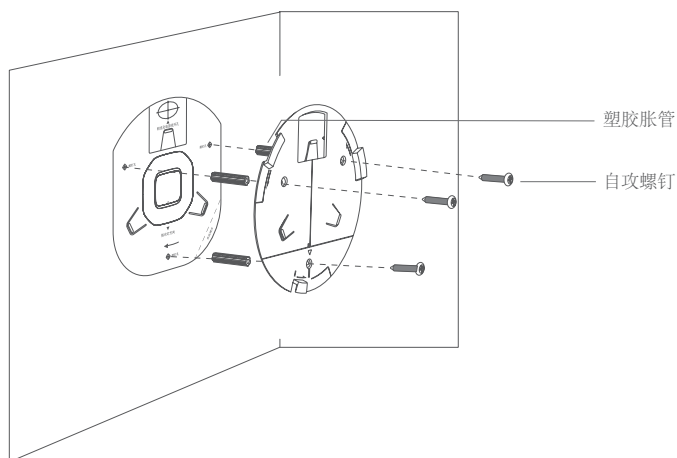
图3-11 固定安装架到墙面示意图
