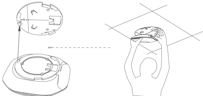
图3-6 安装AP到安装架示意图
