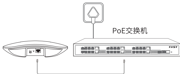
图2-1 PoE供电示意图
