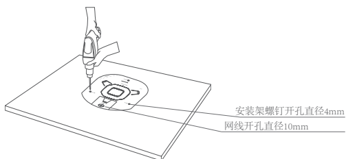
图3-3 钻孔示意图
