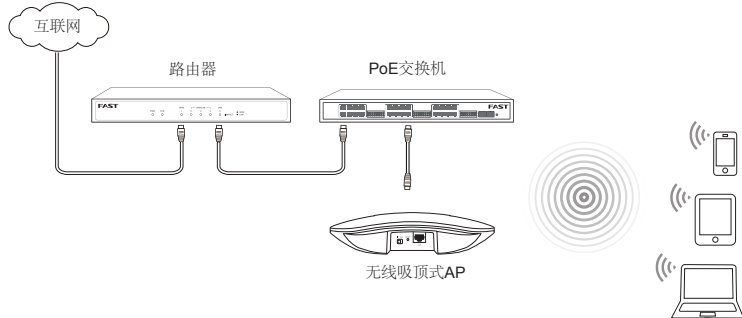
图1-3 典型应用拓扑图-FAT AP模式
